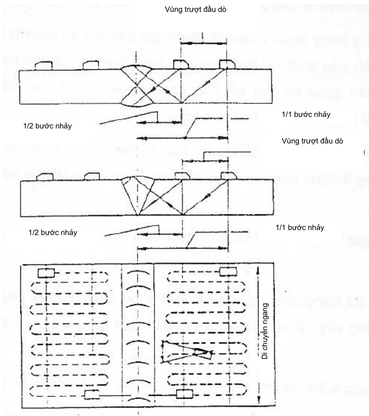
Hình 3 - Hướng di chuyển đầu dò kiểm tra mỗi hàn đối đầu, thiết bị xách tay
