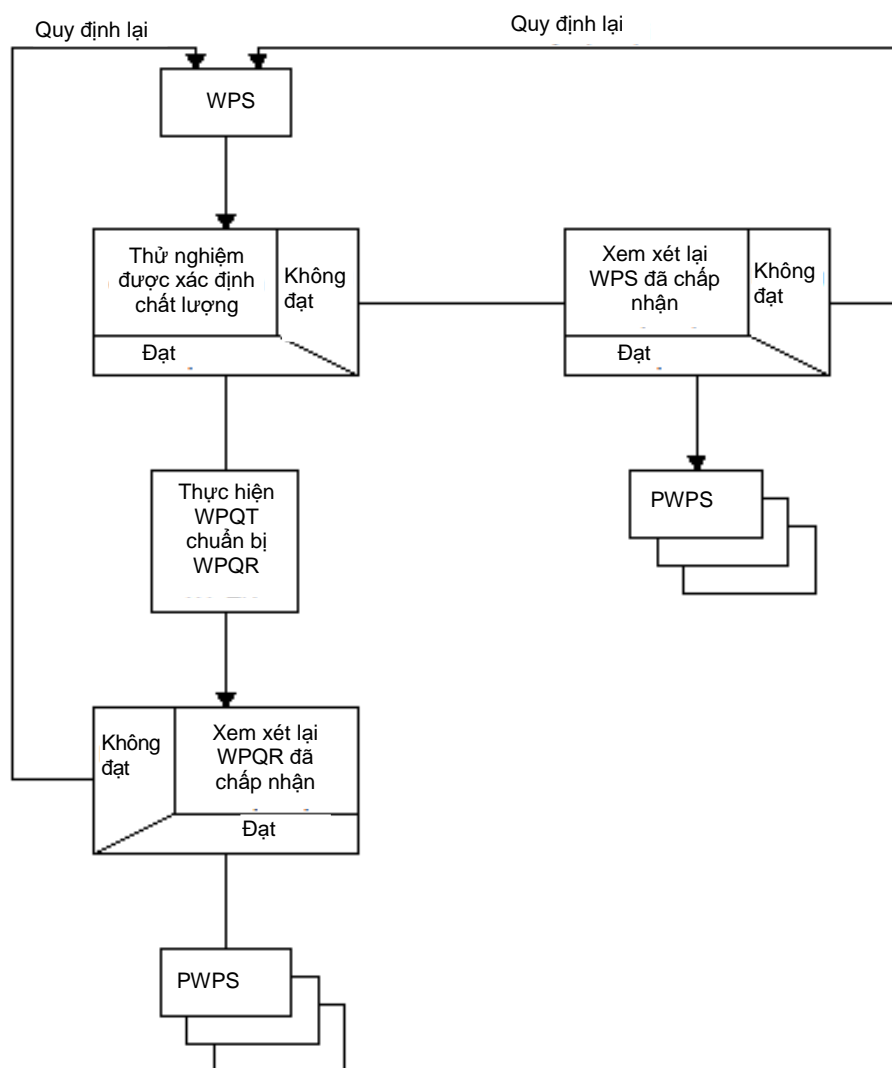
Hình 2 - Sơ đồ các bước chuẩn bị quy định kỹ thuật của quy trình hàn sản xuất
