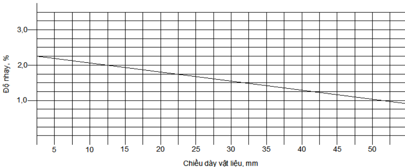
Hình 5 - Đường cong độ nhảy IQI
