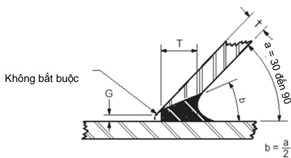
Mặt cắt A-A
